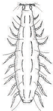
Fig. 7.15: Pauropoda. (CM)
