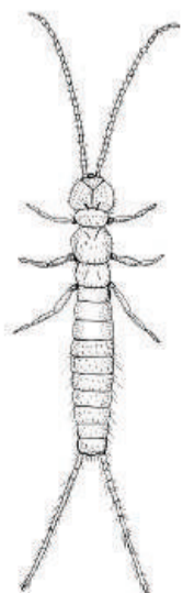
Fig. 7.13: Diplura. (CM)
