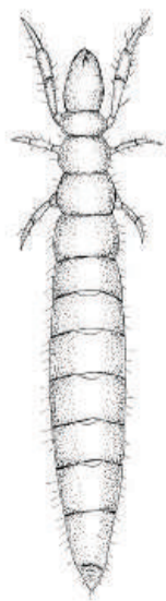
Fig. 7.12: Protura. (CM)
